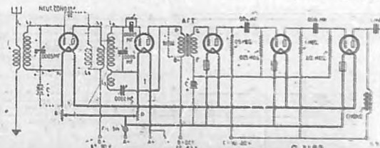
EL RECEPTOR DE CINCO VALVULAS
